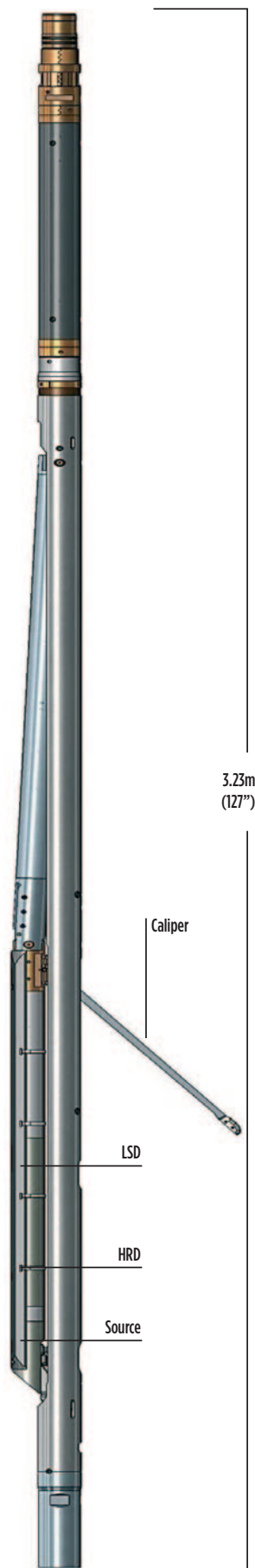
Litho-Density Module
